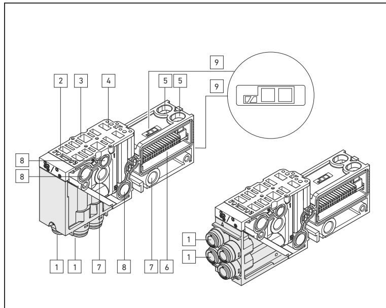
Vista general de la placa base funcional (FGP) con conexiones neumáticas orientadas hacia abajo (izquierda) o en la parte frontal (derecha)
