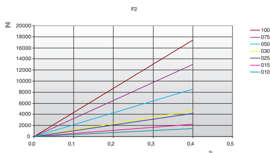
Carico / Allungamento [%]
